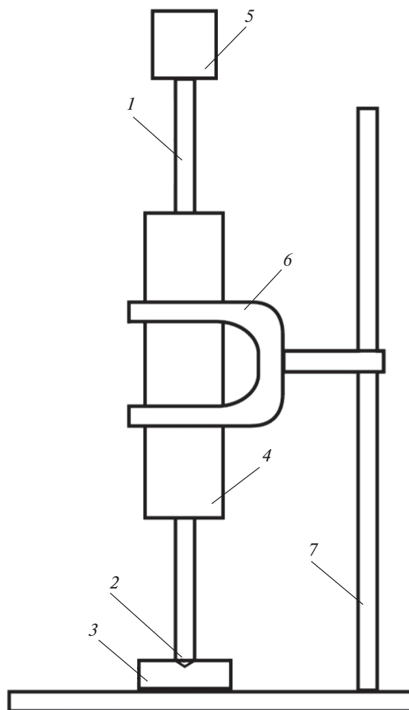
Рис. 1. Схема специального стенда для отбора вещества с упругой поверхности твердого тела. 1 — пробоотборник в виде кварцевой трубочки с торцевой шероховатой поверхностью на торце; 2 — место контакта шероховатой поверхности пробоотборника с упругой поверхностью анализируемого тела; 3 — упругое твердое тело; 4 — вертикальное направляющее устройство; 5 — грузик, создающий контролируемое давление на поверхность анализируемого тела; 6 — держатель направляющего устройства; 7 — штатив.
